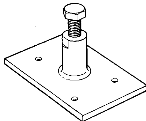
Y.20532 Ausbauwerkzeug Kurbelwelle Outil de démontage du vilebrequin Dismounting tool crankshaft
