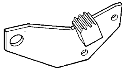
Y.20542 Sicherung für Zahnräder Arrêt pour engrenages Gear blocking tool
