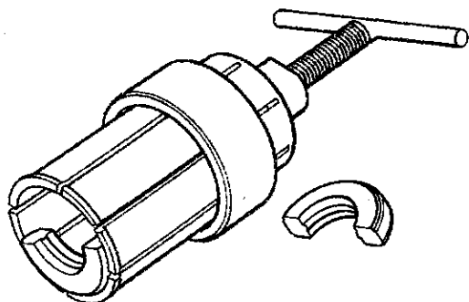
Y.20546 Halbschalen für Abziehen T0011449 Demi-coquilles pour outil d'extraction T0011449 Shells for extractor T0011449
