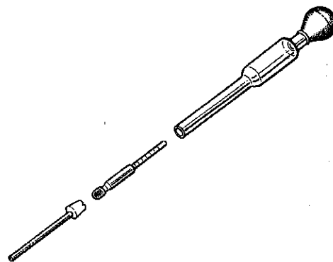
Y.20564 Dichtemesser für Kontrolle Batterieladezustand Densimètre de contrôle charge-batterie Battery charge densimeter
